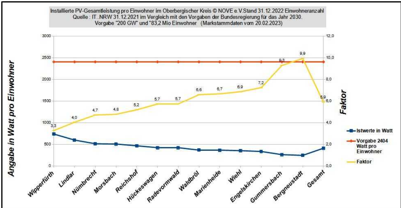
Bild 3. Installierte PV-Gesamtleistung im OBK pro Einwohner mit Zielvorgabe Stand 31.12.2022
