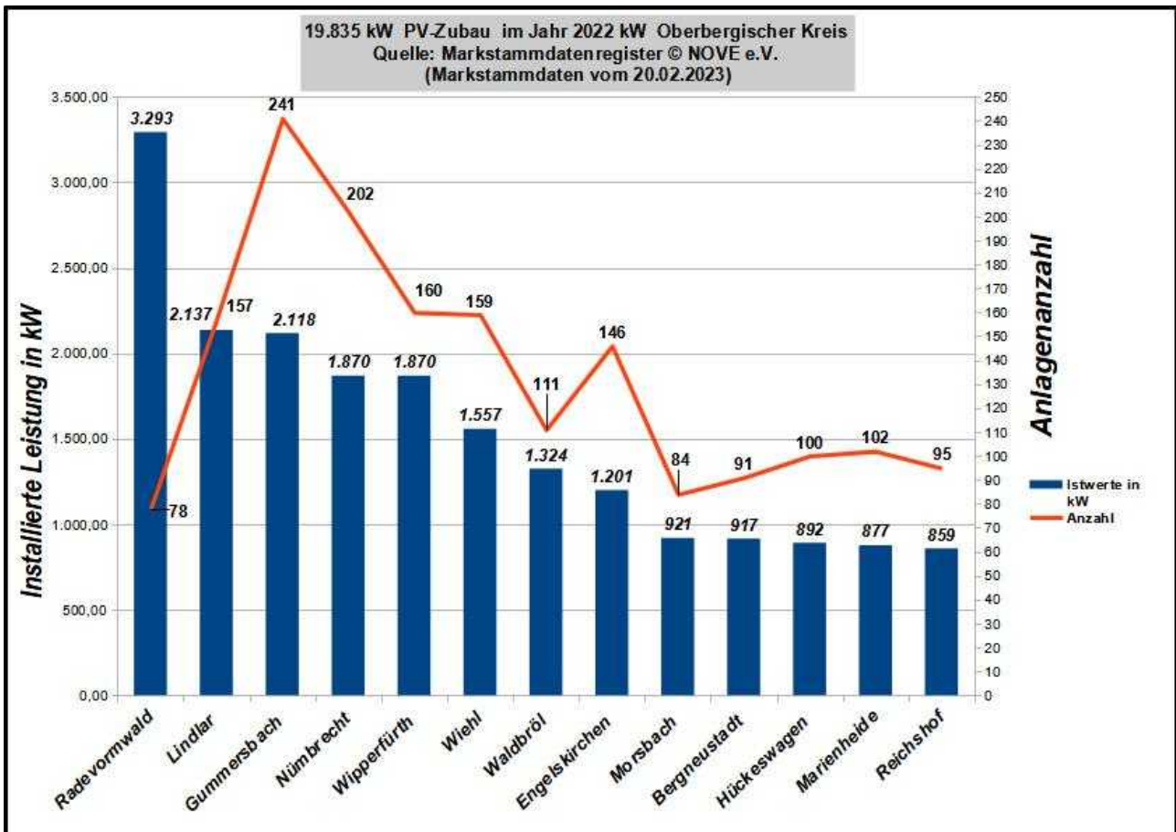
Bild 4. Zubau für 2022 aufgeschlüsselt nach Kommunen
