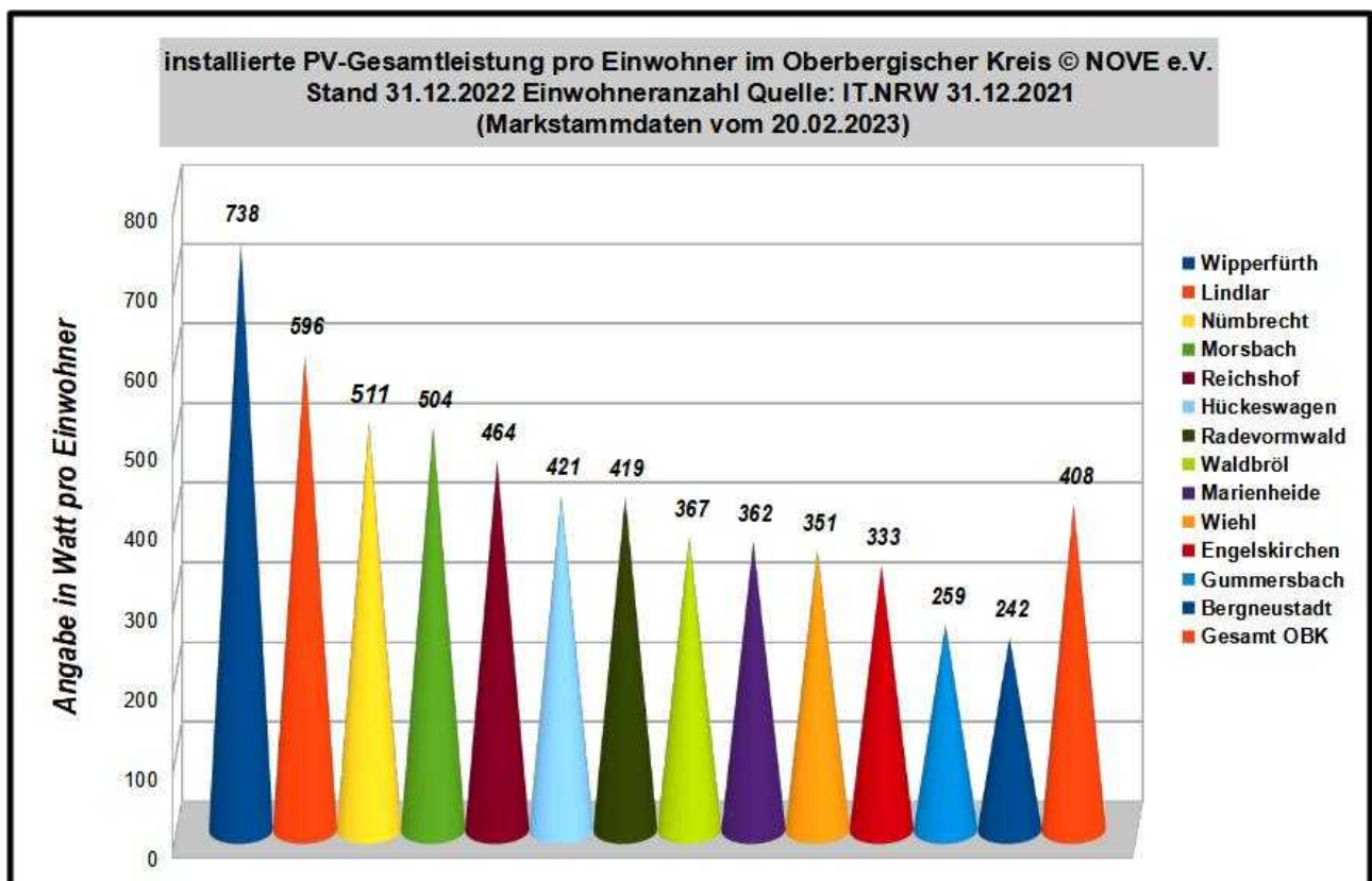
Bild 2. Installierte PV-Gesamtleistung im OBK pro Einwohner Stand 31.12.2022
