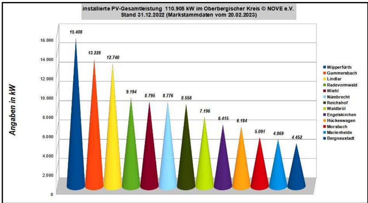
Bild 1. Installierte PV-Gesamtleistung im OBK Stand 31.12.2022
