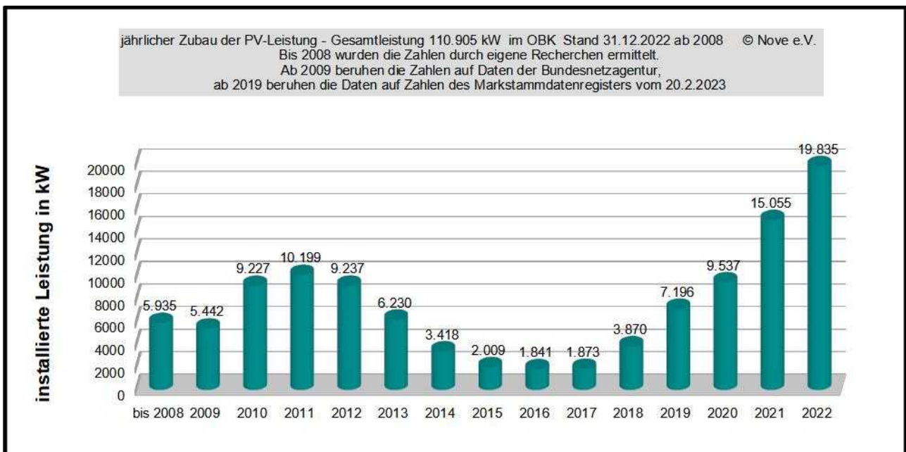
Bild 4. jährlicher Zubau ab 2008 bis 2022
